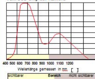
Spektralempfindlichkeitskurve vom CCD-Chip der Kamera
