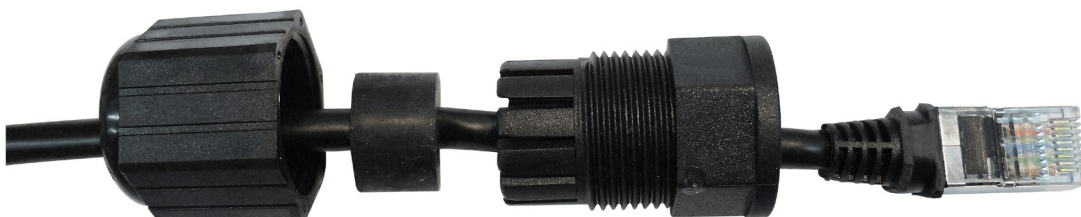
Abbildung 4 Das Gegenstück nun über den Stecker einsetzen und Gummidichtung nach oben in die Zahnung schieben.
