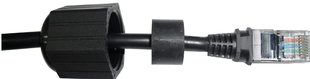
Abbildung 3 Überwurfmutter und Gummidichtung (Dichtung ist auf einer Seite offen) über den Stecker einsetzen
