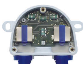
MX-Overvoltage-Protection-Box-RJ45: MOBOTIX-Patchkabel auf MOBOTIX-Patchkabel
