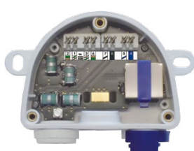
MX-Overvoltage-Protection-Box-LSA: MOBOTIX-Patchkabel auf Netzwerk-Verlegekabel
